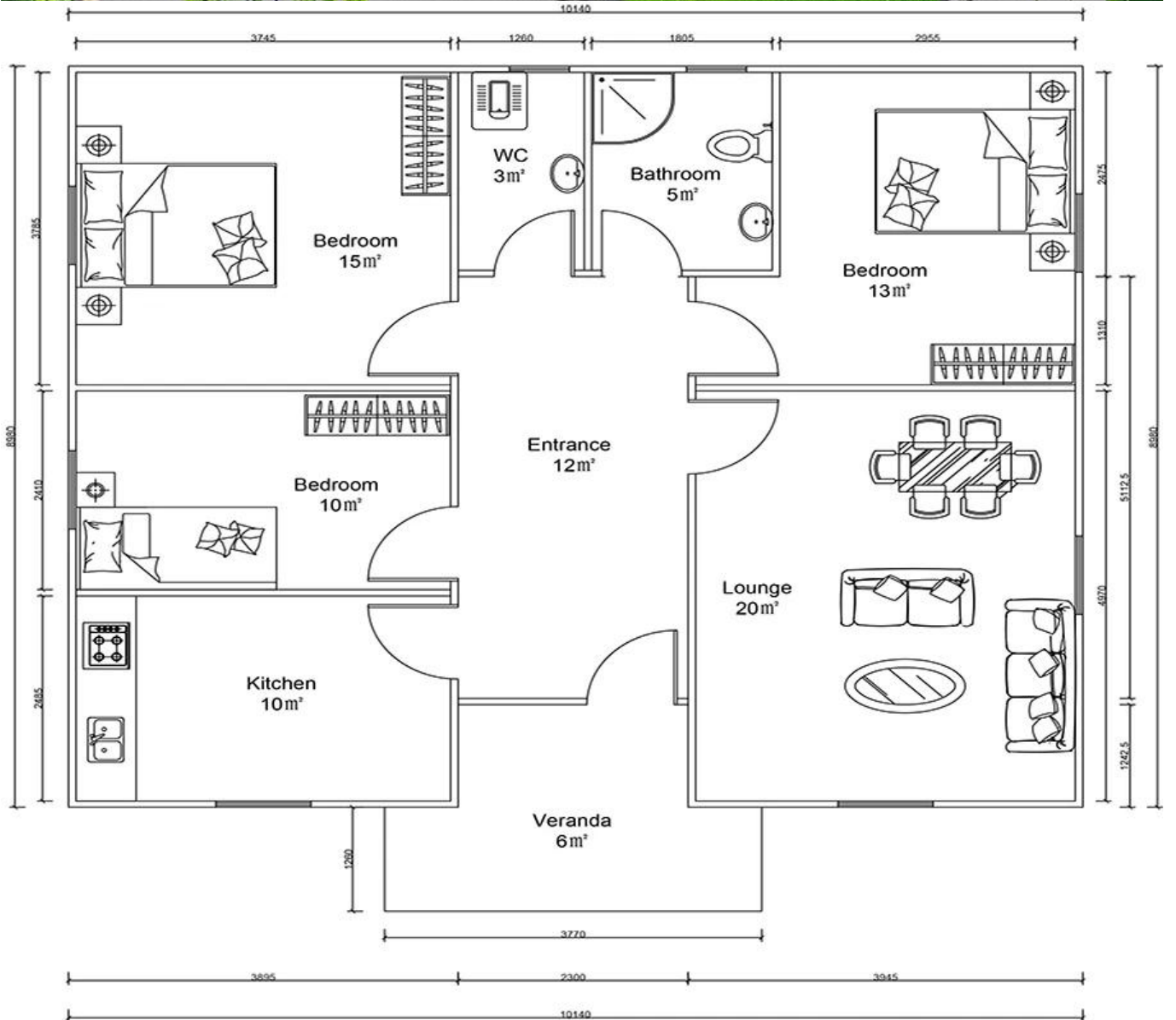
Prefabrik ev detayları
